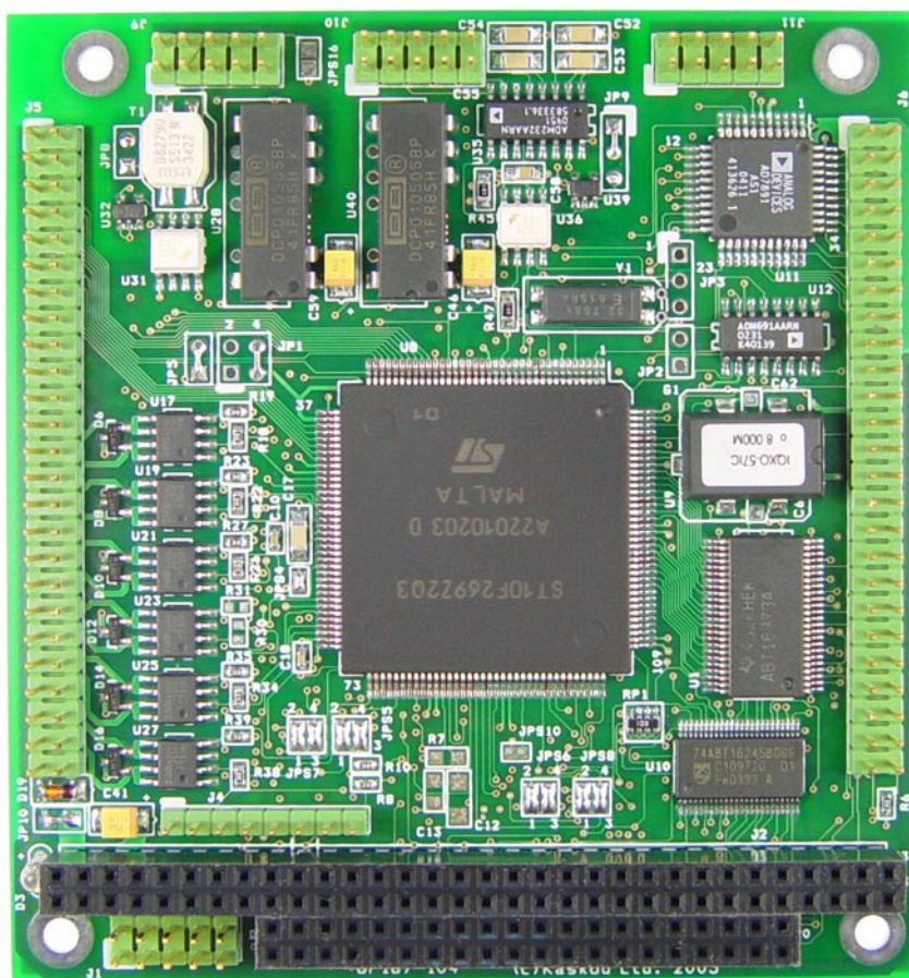
Рис. 1 Внешний вид контроллера GP269-104
