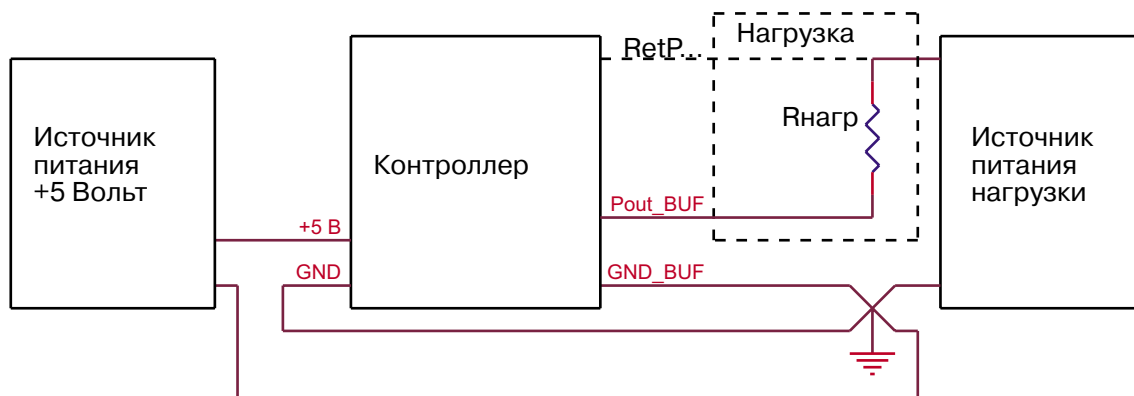
Рис. 6 Структурная схема подключения источников питания и нагрузок.
