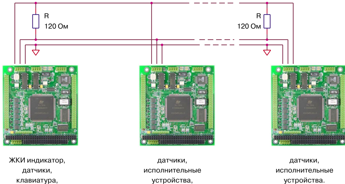
Рис. 3 Подключение контроллера к CAN-сети
